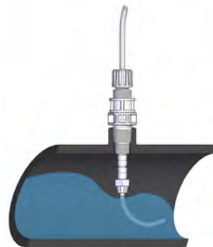
INSTALLATION 1/2" EXTENSION AVEC FLEXIBLE ANTI CRISTALLISATION INSTALLATION ON 1/2" WITH ANTI FOAL FLEXIBLE EXTENSION
