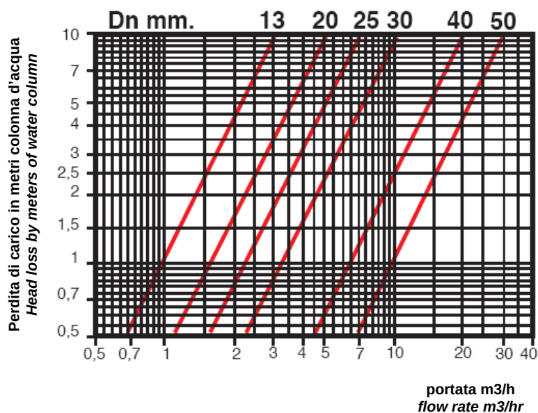
DIAGRAMMA DELLE PERDITE DI CARICO HEAD LOSS DIAGRAM
