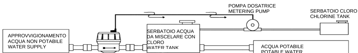
APPLICAZIONI PER CONTATORI EQUIPAGGIATI CON EMETTITORE D'IMPULSI APPLICATION EXAMPLES
